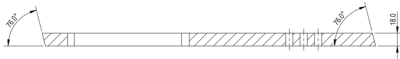
SECTION A-A SCALE 1 : 3
