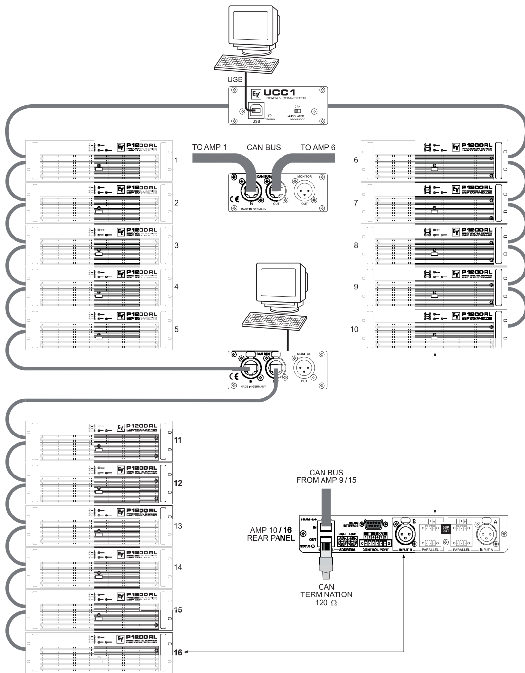
System mit mehreren Racks und mehreren UCC1 / PCs
